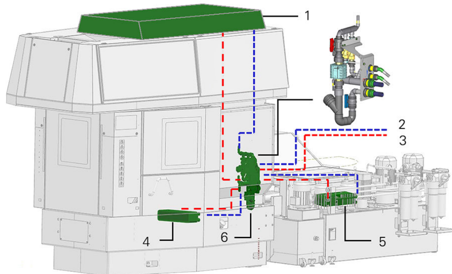
Beispiel: Schema Kühlung MS
