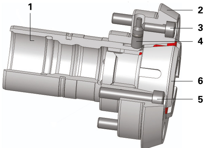
Exemple : Tête de serrage du système Spanntop (marque Hainbuch)
