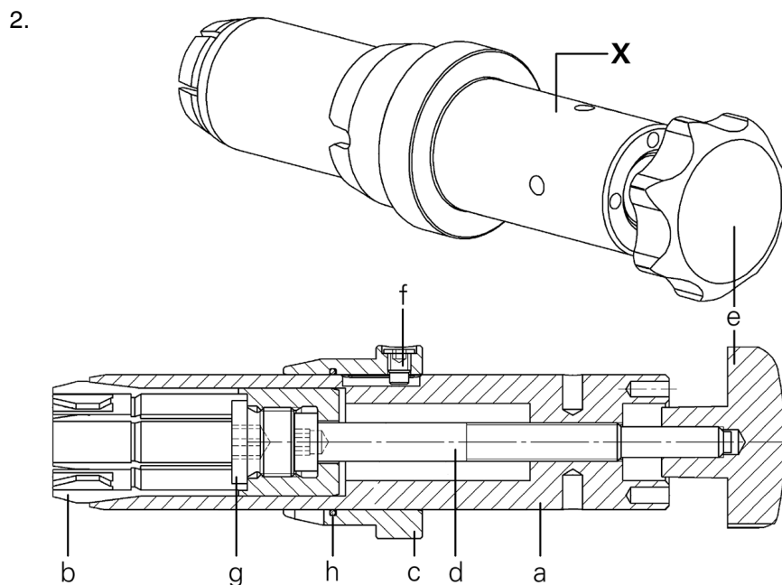
Exemple : Dispositif de changement (clé RS) des pinces d'avance MS16-6 (marque Hainbuch)
