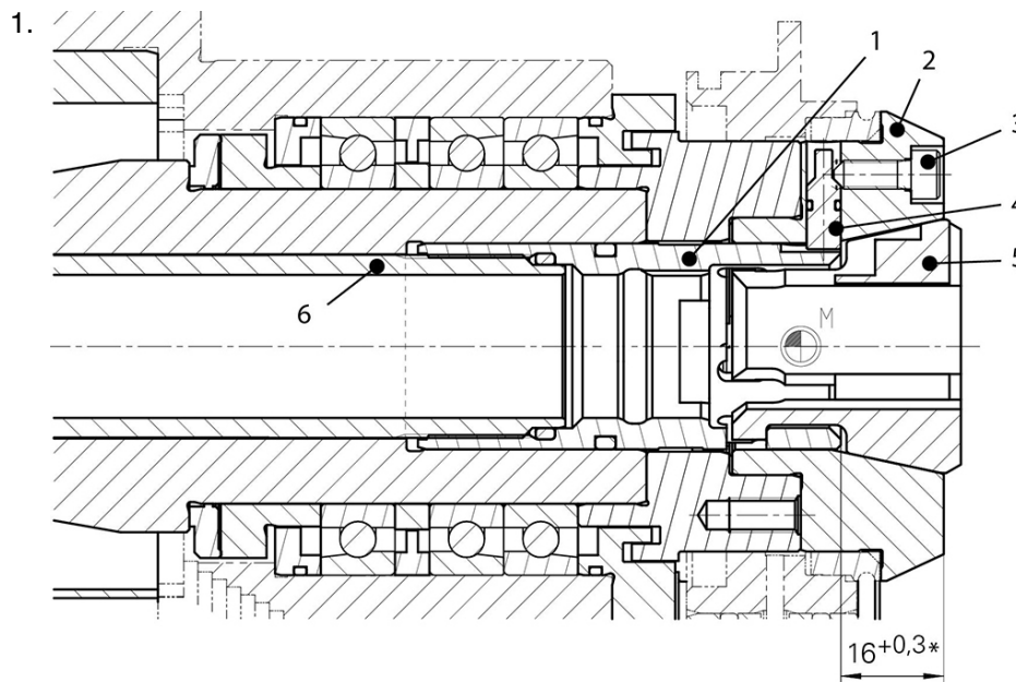
Exemple : Système de serrage MS16-6 Plus (marque Hainbuch) Spanntop
