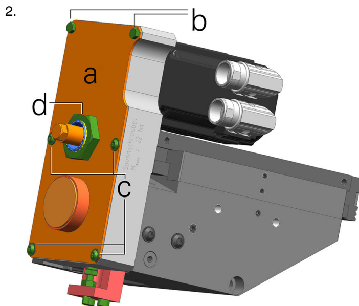
Entraînement par courroie dentée du MS16-6 5 6 01
