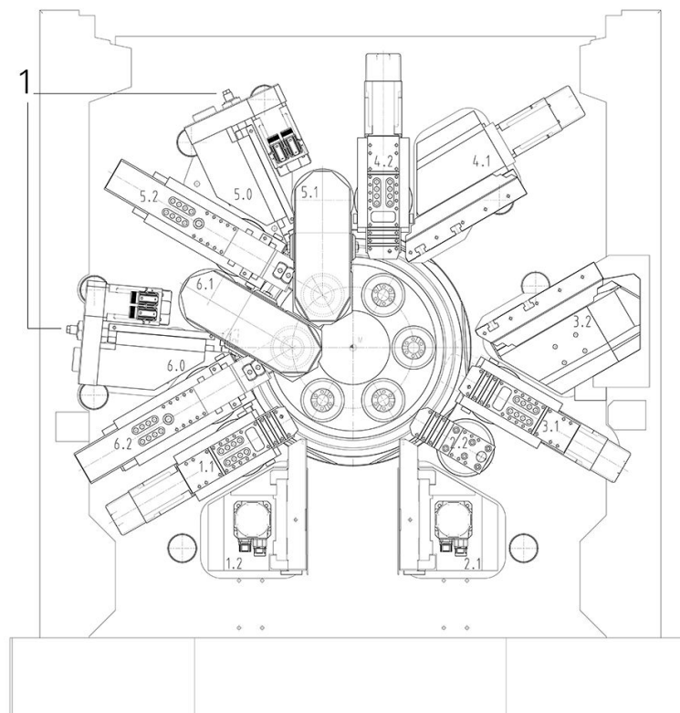
Entraînement à courroie MS16-6 (1 – chariots 5.0 et 6.0)
