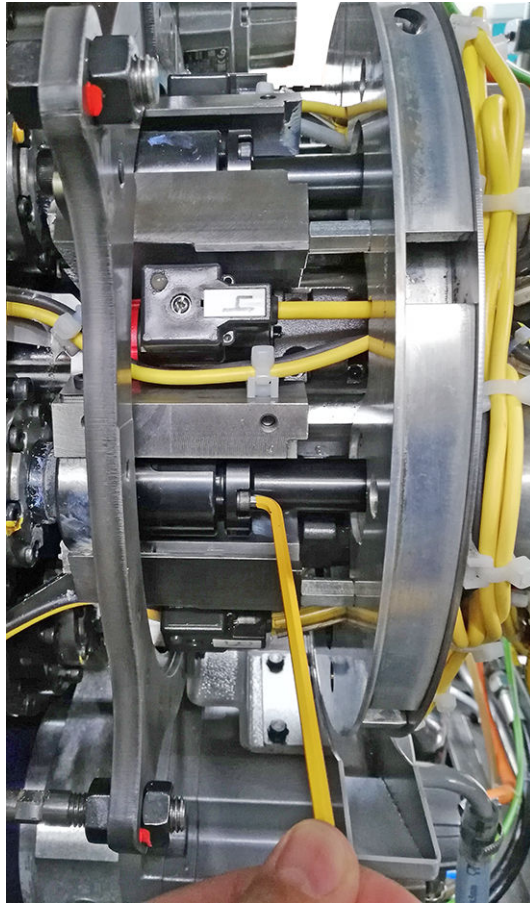
Exemple : Figure 1 : Desserrer les 3 vis au dos des broches
