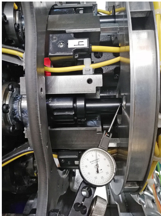
Exemple : Figure 2 Contrôler la rotondité
