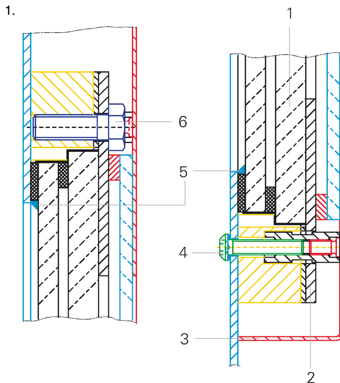
Exemple : Vitre d'observation MS22-6/MS22-8/MS32-6.2/MS40-6
