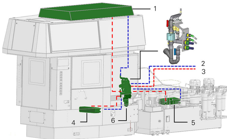
Exemple : Schéma du refroidissement MS
