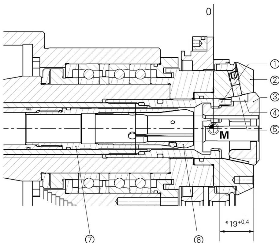
Exemple : Système de serrage MS16-6 (marque Hainbuch) SPANNTOP
