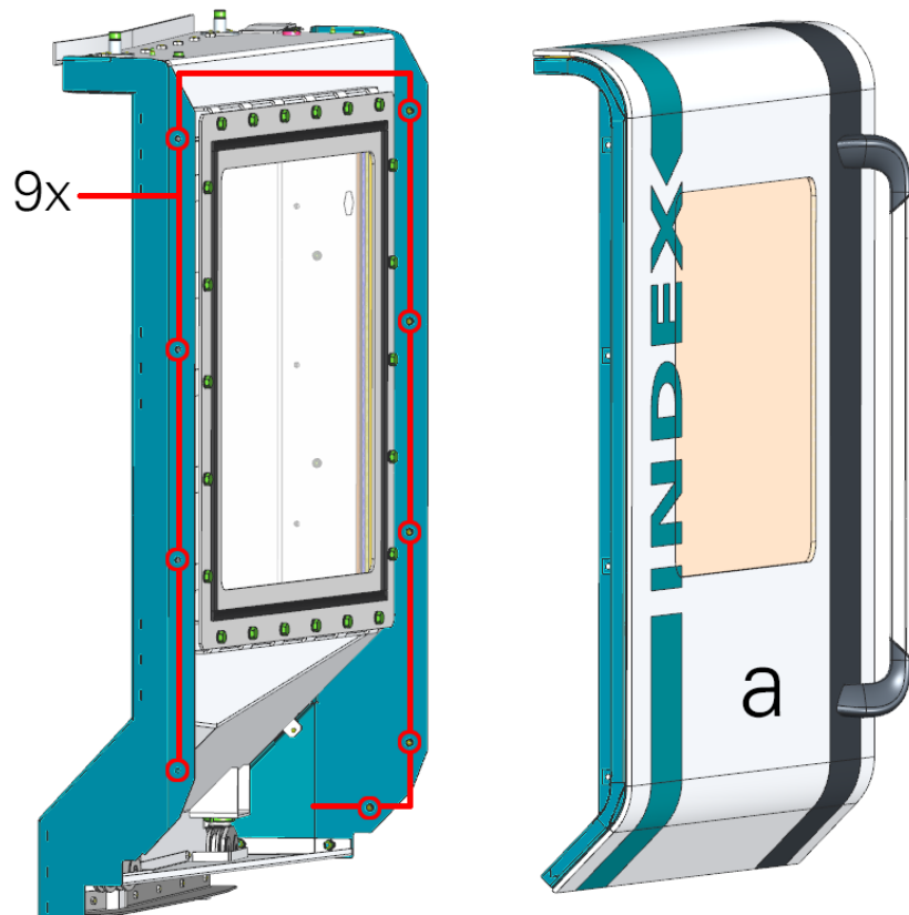
Beispiel: MS32-6.3 Sichtscheibe Arbeitsraumbtuer 2 (Abb. 3)
