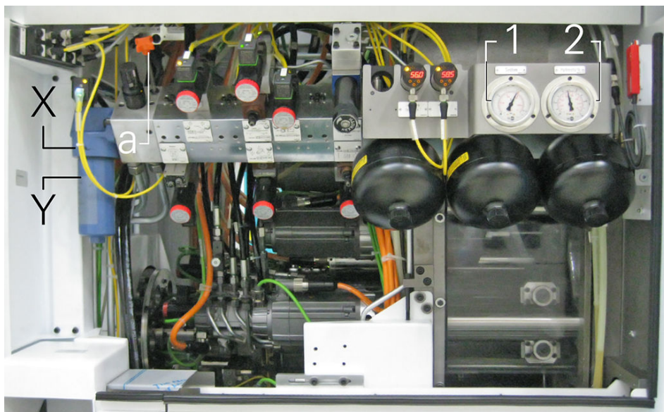
Exemple : Groupe hydraulique MS32-6.3
