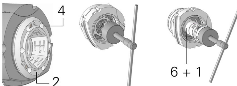
Exemple : Démonter le logement d'élément de serrage et le corps de base
