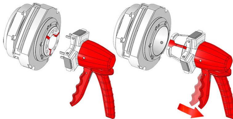
Exemple : Extraire_la_pince_de_serrage (marque Hainbuch)
