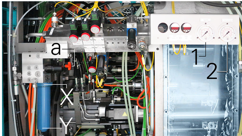
Exemple : Groupe hydraulique MS52-6.3
